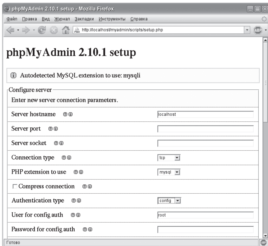
Рис. 7.4. Определение параметров настройки соединения с сервером MySQL
