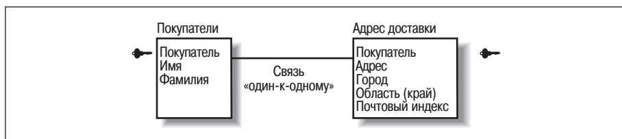
Рис. 8.1. Связь «один-к-одному» между покупателями и их адресами
